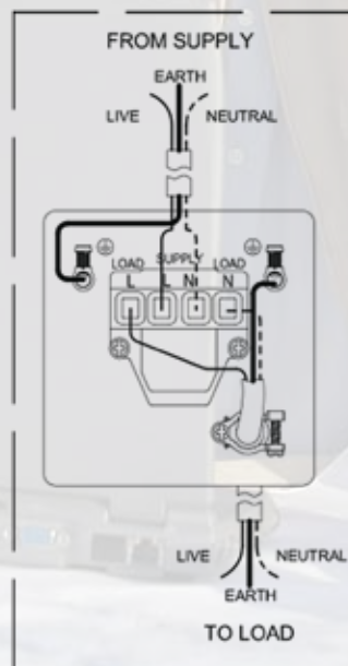
20A SWITCH
