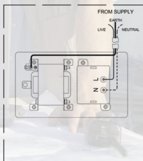
SHAVER SOCKET
